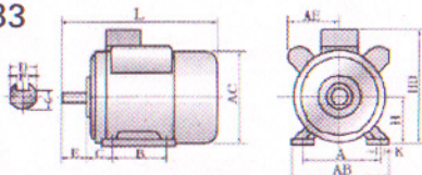
IMB3
