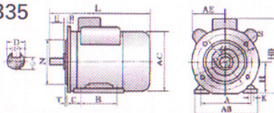
IMB35
