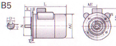
IMB5
